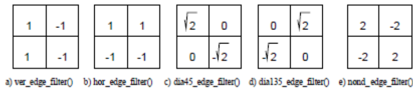
Figure 3 – Filtros 2x2 para detecção de fronteiras
