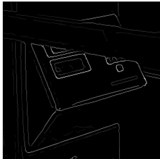
Edge Detection
