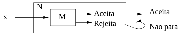
Figura 13: Construção da máquina N
