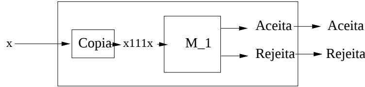
Figura 12: Construção de M' que aceita L_d
